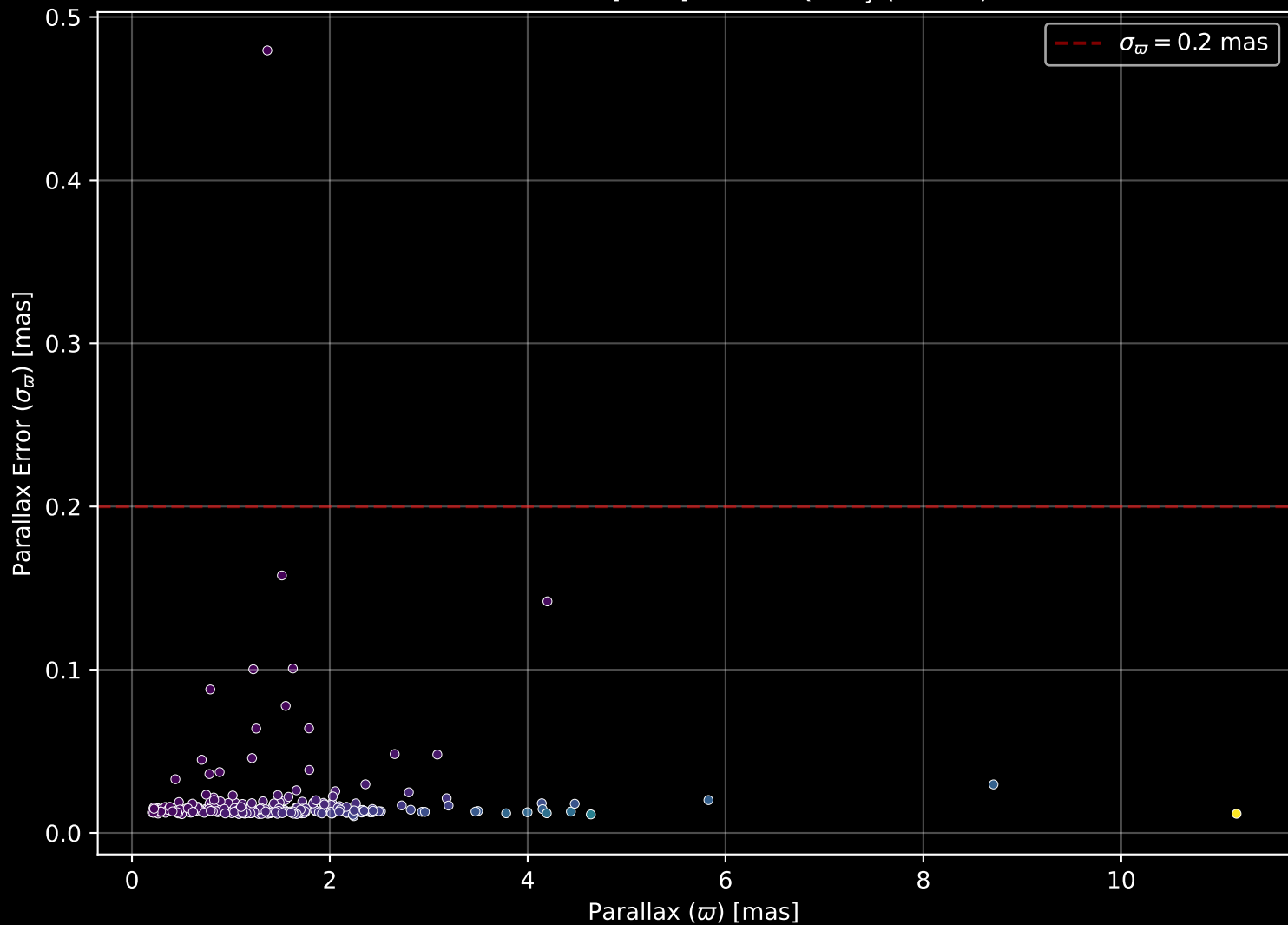
GALAH DR4 Field: [1857] Parallax Quality (n= 254)
