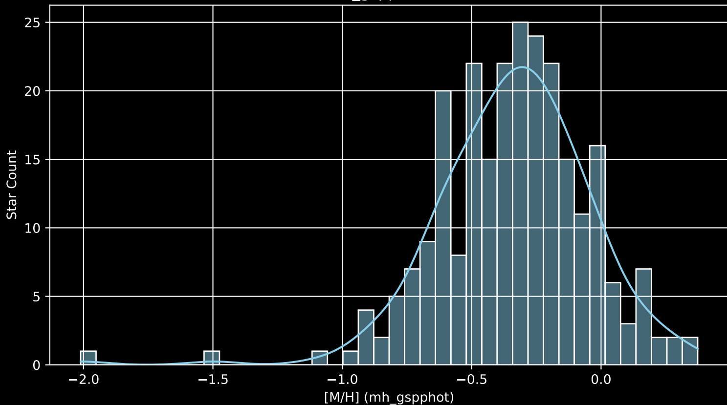
GALAH DR4 Field: [1857] [M/H] (mh_gspphot) (n= 253)
