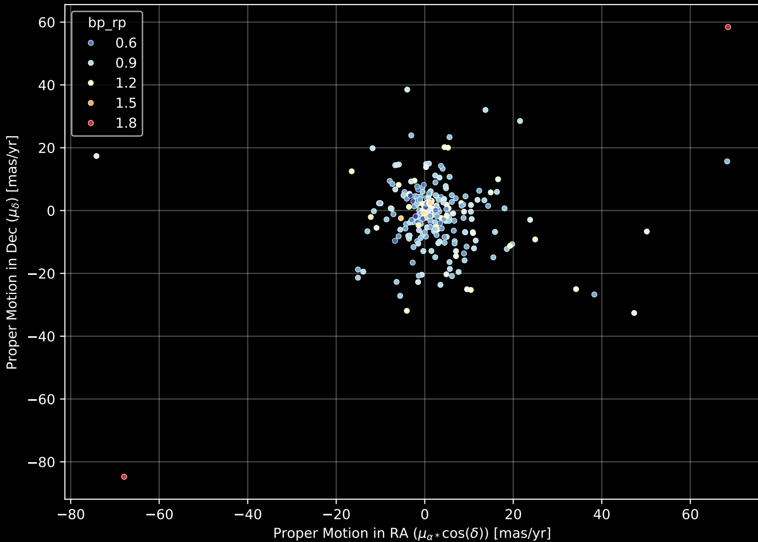
GALAH DR4 Field: [1857] Proper Motion Diagram (n= 254)
